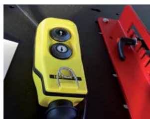
Pulsantiera a cavo con magnete e predisposto per il montaggio del kit radiocomando wifi LV8 Wire remote control unit with magnet and arranged for assembling the LV8 wi-fi remote control kit
